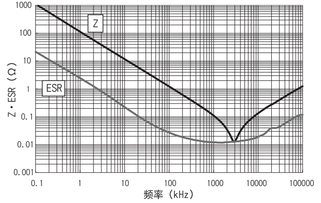
●KVF 系列 50V / 1.0μF
