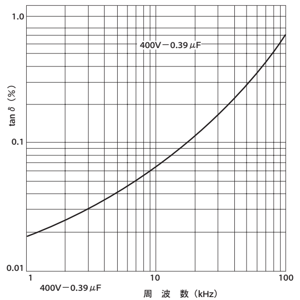
誘電正接 (tan \delta ) - 周波数特性 (at 20°C)
