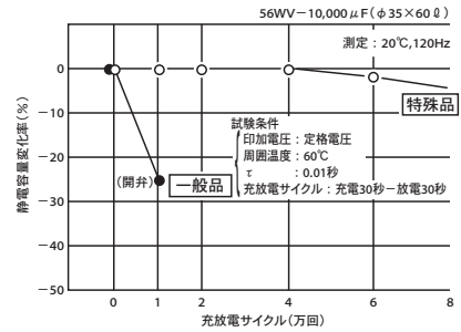
Fig-23 急充放電特性 (充放電回数の影響)
