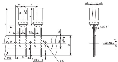
Fig.4 テーピングコード TE \phi 12.5
