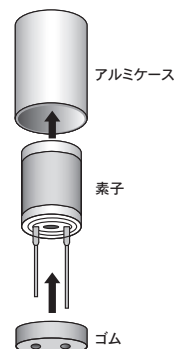
含浸概略図
