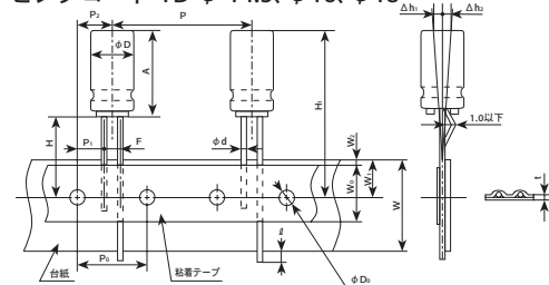
テーピングコード TD \phi 14.5, \phi 16, \phi 18
