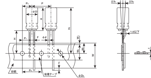
Fig.3 テーピングコード TD \phi 6.3 ~ 12.5
