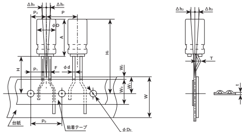
Fig.1 テーピングコード TX \phi 5
