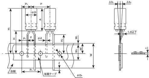
Fig.3 テーピングコード TD \phi 6.3 ~ 12.5
