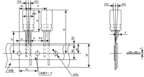
Fig.2 テーピングコード TD \phi 6.3 \sim 10
