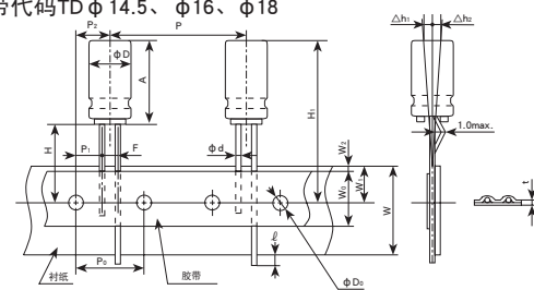
Fig.4 编带代码TE \phi 12.5 编带代码TD \phi 14.5 、 \phi 16 、 \phi 18
