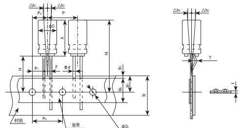
Fig.2 编带代码 TD \phi 6.3 \sim 10
