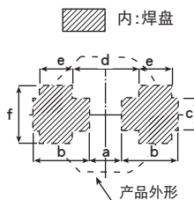
Fig.3 铸模贴片型 (与7343尺寸通用)
