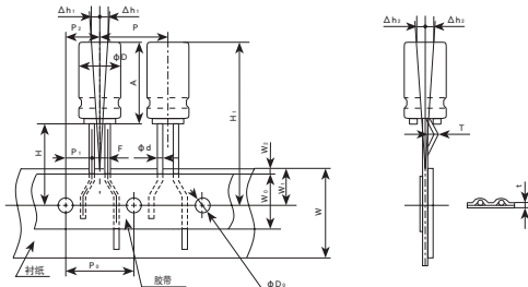
Fig.1 编带代码 TX \phi 5
