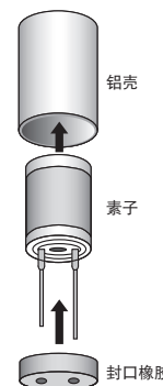
含浸概略图
