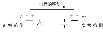
图22: 放电时的电荷状态 (断开电源V1, 放电后的状态)
