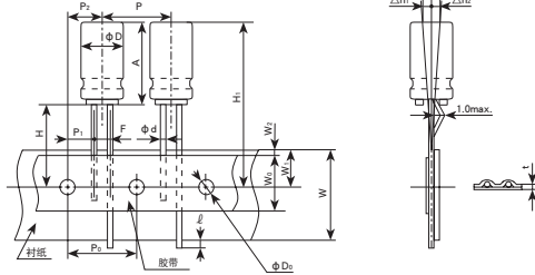
Fig.3 编带代码TD \phi 6.3 \sim 12.5
