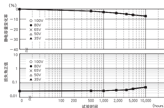
图20: 耐久性(电压参数)
