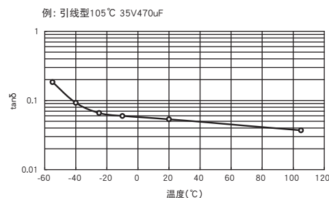
图11: \tan \delta 的温度特性
