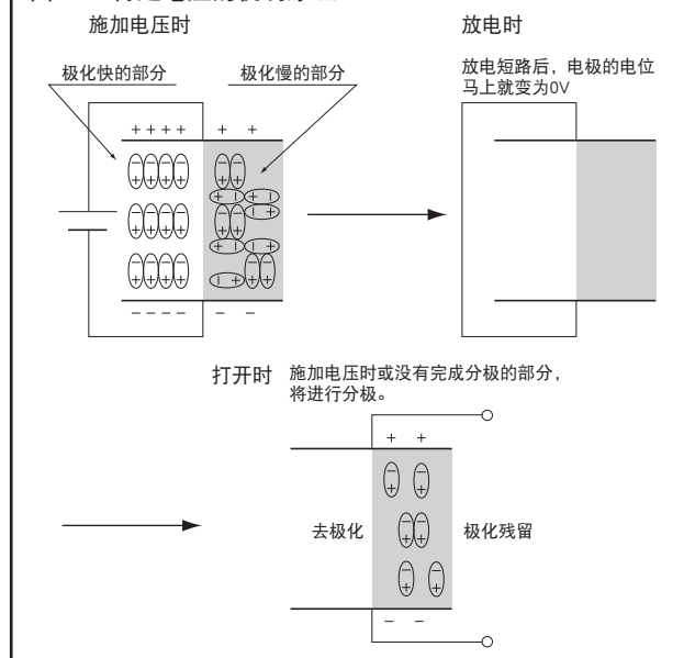
图28：再起电压的机制原理
