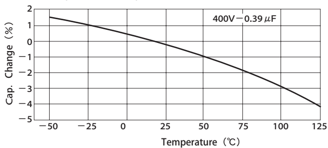
1 kHz Capacitance-Temperature
