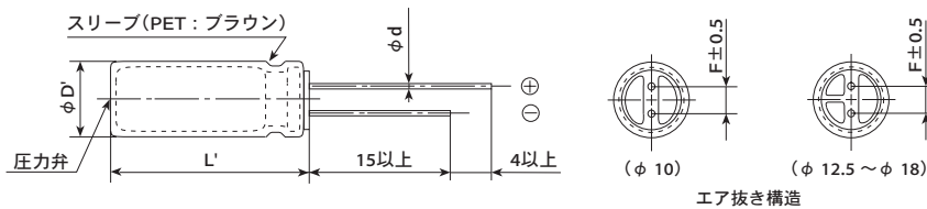
エア抜き構造
