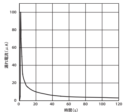
Fig-12 漏れ電流の時間的変化
