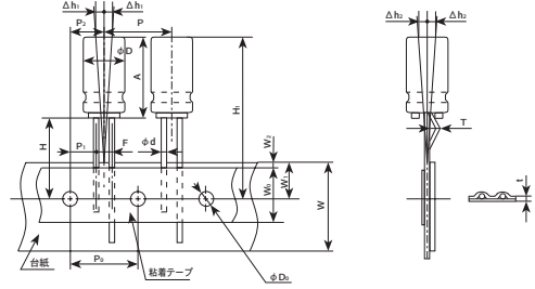
Fig.2 テーピングコード TD φ 6.3~10
